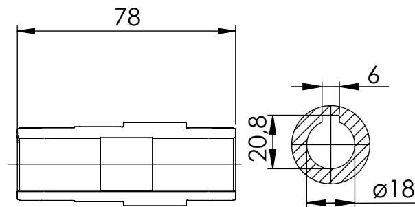
Detalhe eixo de saída Outup shaft detail Detalle del eje salida (Sem escala/no scale/sin escala)
